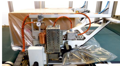
4- Nahtschweissung
